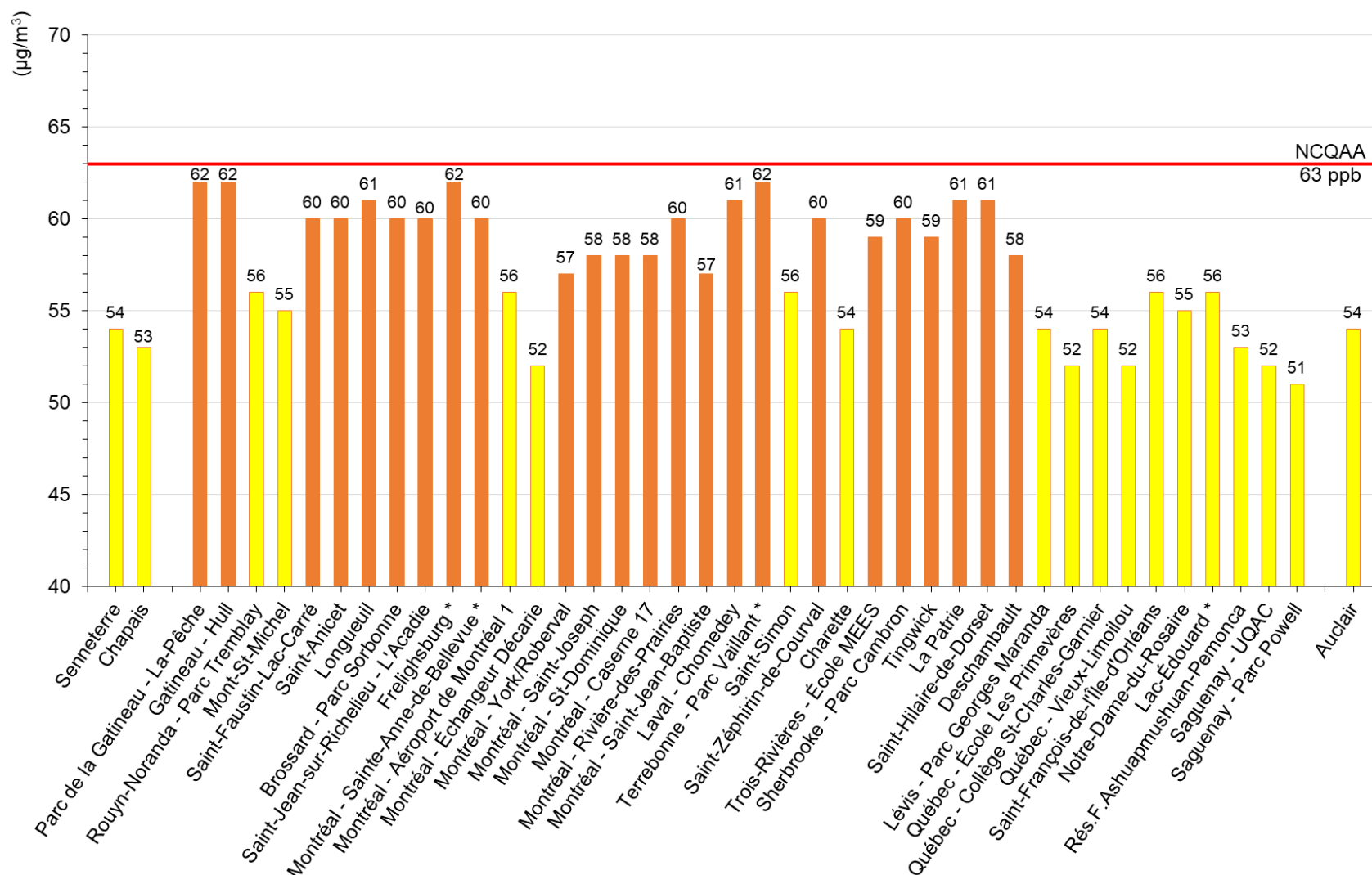
Figure 4 Concentrations d'ozone sous la forme statistique de la NCQAA pour la période 2016-2018
