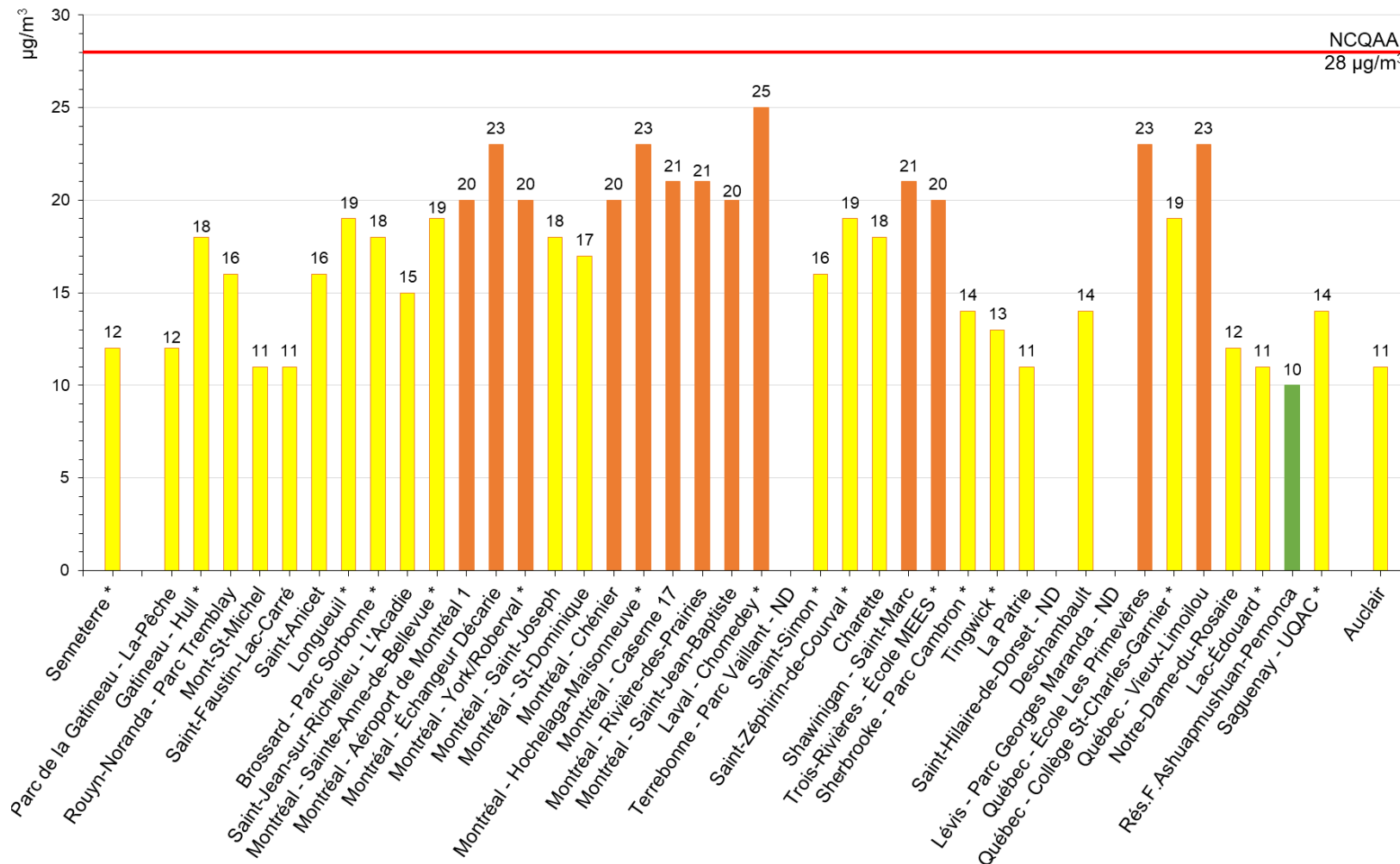
Figure 2 Concentrations de particules fines sous la forme statistique de la NCQAA (24 heures) pour la période 2016-2018
