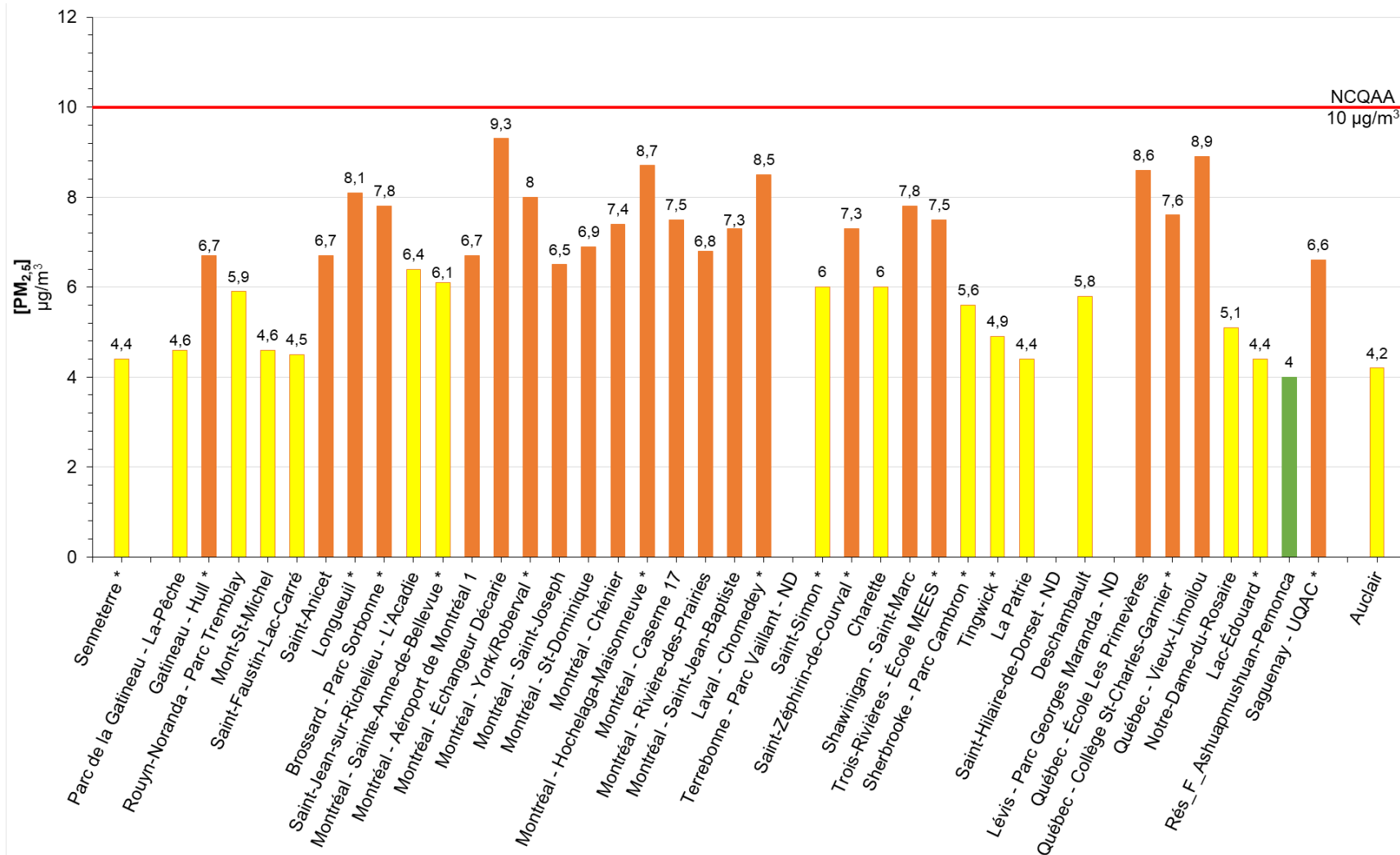
Figure 3 Concentrations de particules fines sous la forme statistique de la NCQAA (année civile) pour la période 2016-2018
